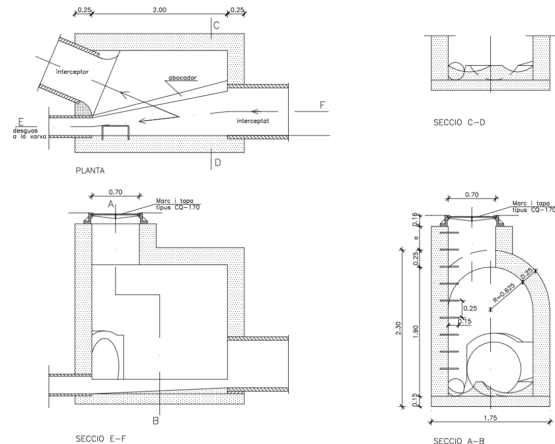
SOBREEIXIDOR TIPUS, SECCIONS NO VISITABLE
