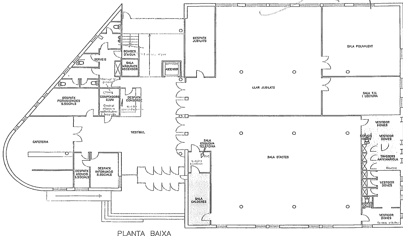
PLANTA BAIXA
